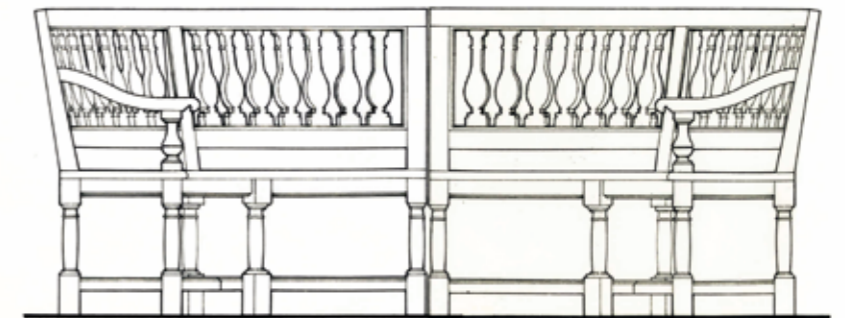
33 pouces (84,3) ÉLÉVATION VUE DE FACE (2 bancs en quart de cercle à 6 pieds chacun)
