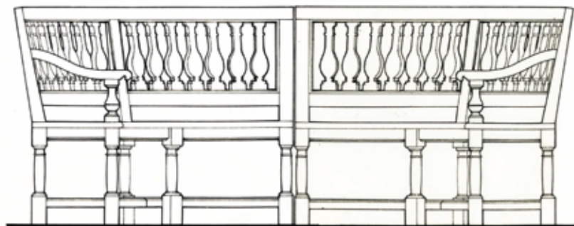
12 places (60,5) ÉLEVATION VUE DE FACE (2 bancs en quart de cercle à 6 pieds chacun)
