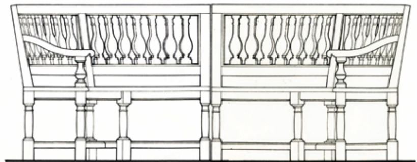
12 places (60,3) ÉLEVATION VUE DE FACE (2 bancs en quart de cercle à 6 pieds chacun)
