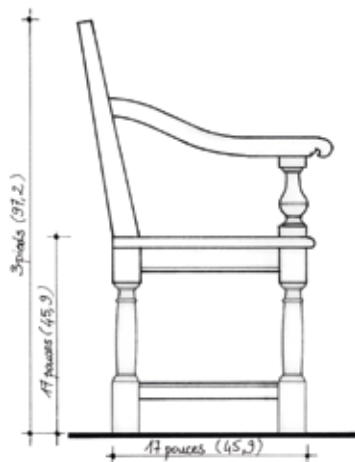
VUE DE PROFIL
